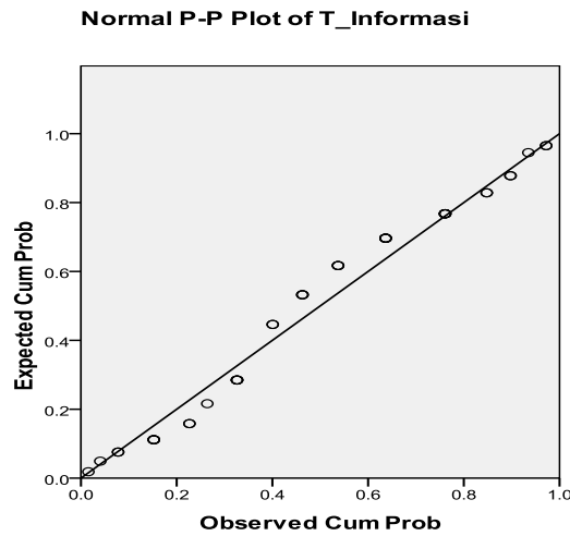
Gambar 1. Grafik Uji Normalitas
