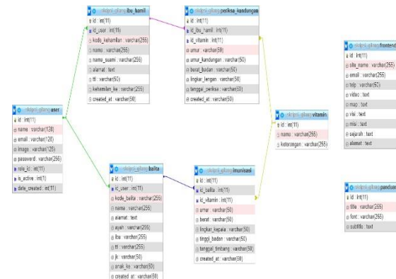
Gambar 2. Rancangan Relasi Tabel
